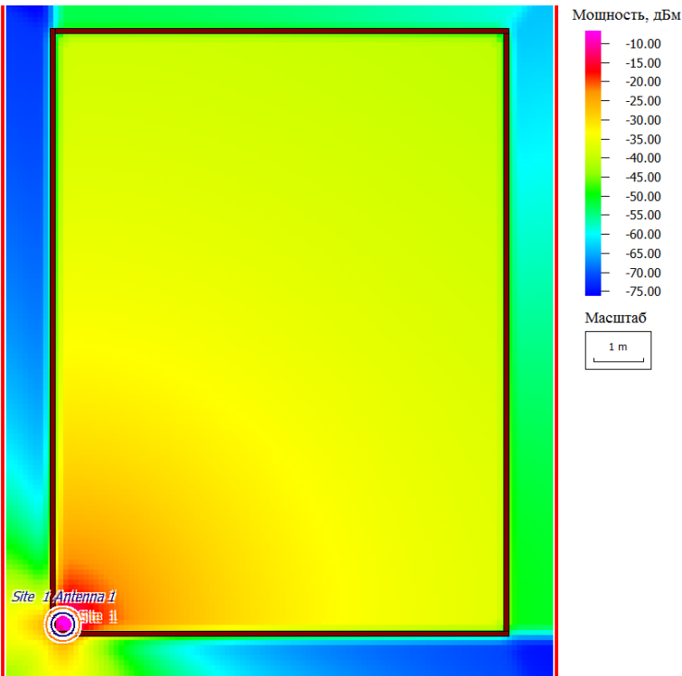
Рисунок 3 – визуализация уровней мощности в исследуемом помещении при частоте 5 ГГц
