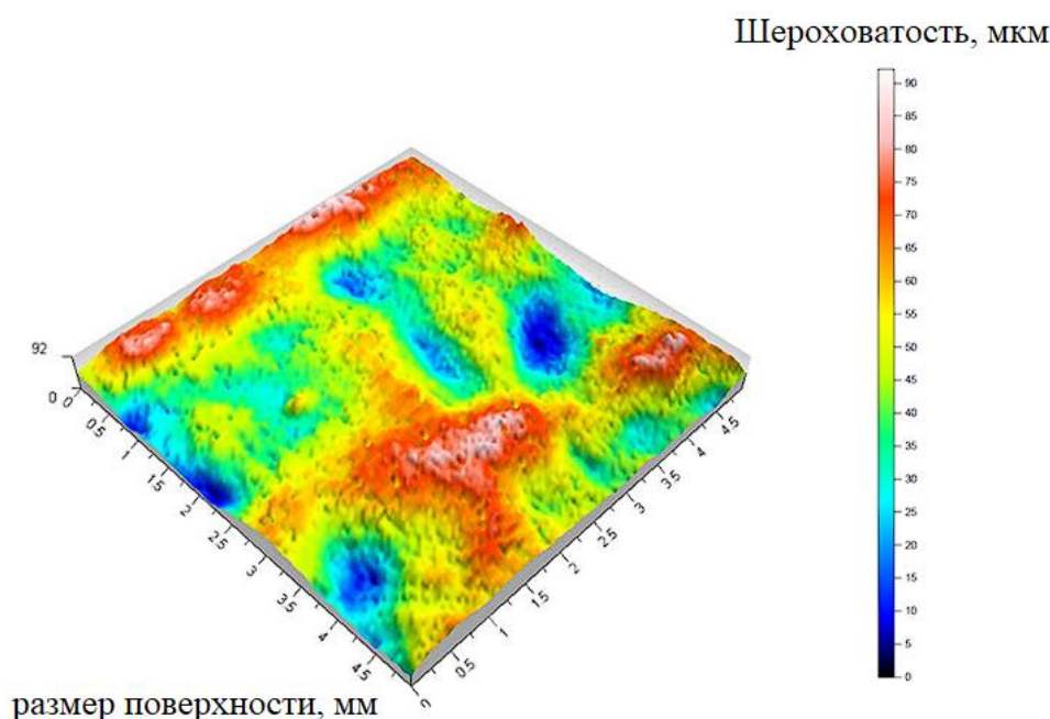
Рисунок 2 – значения шероховатости для куска гипсокартона
